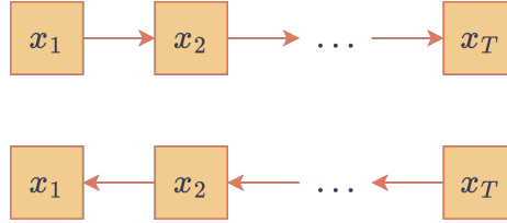
Figura 11: DAGs asociados a un modelo de difusión.
