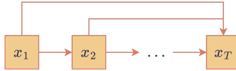
Figura 8: DAG asociado a un modelo autorregresivo.
