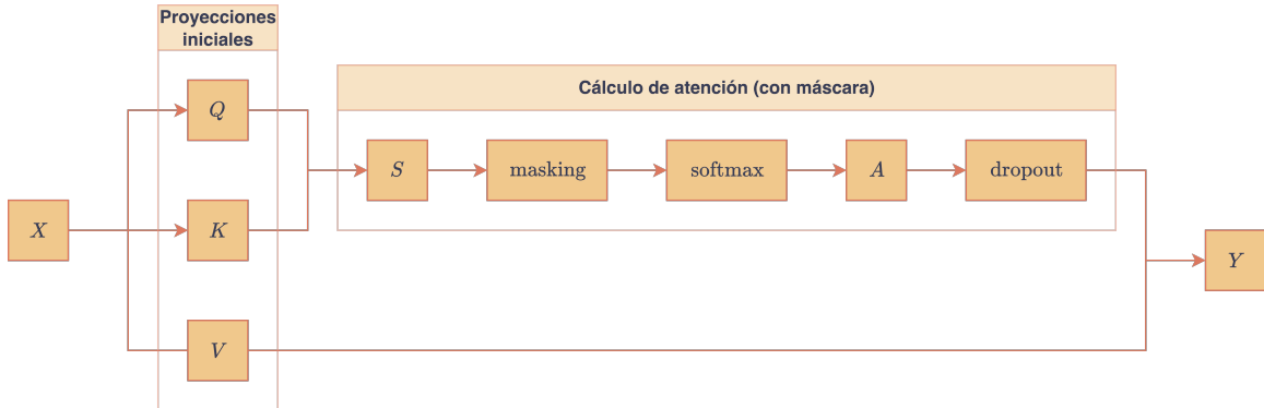
Figura 45: Diagrama del mecanismo de masked self-attention con máscara causal y dropout sobre la matriz de atención.
