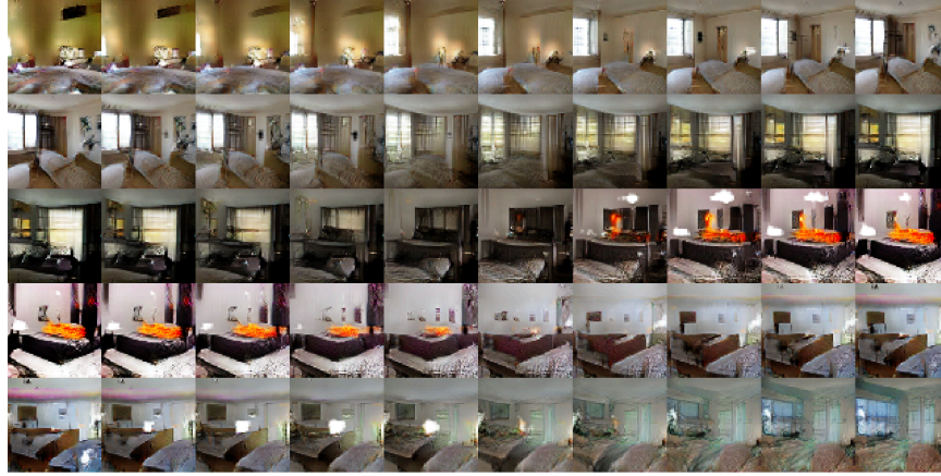
Figura 36: Interpolación latente usando una DCGAN. Imagen obtenida desde [44].
