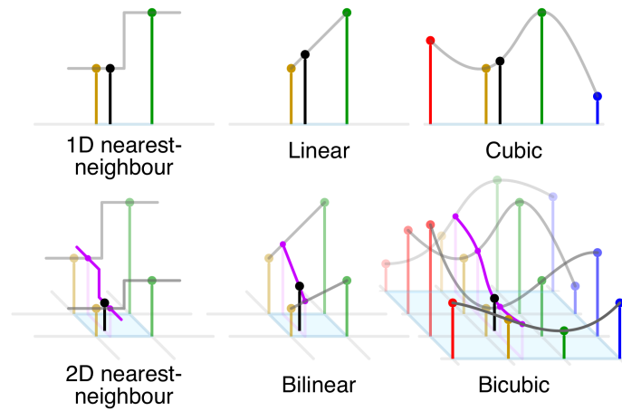
Figura 63: Comparación de interpolaciones en los casos D = 1 y D = 2 .
