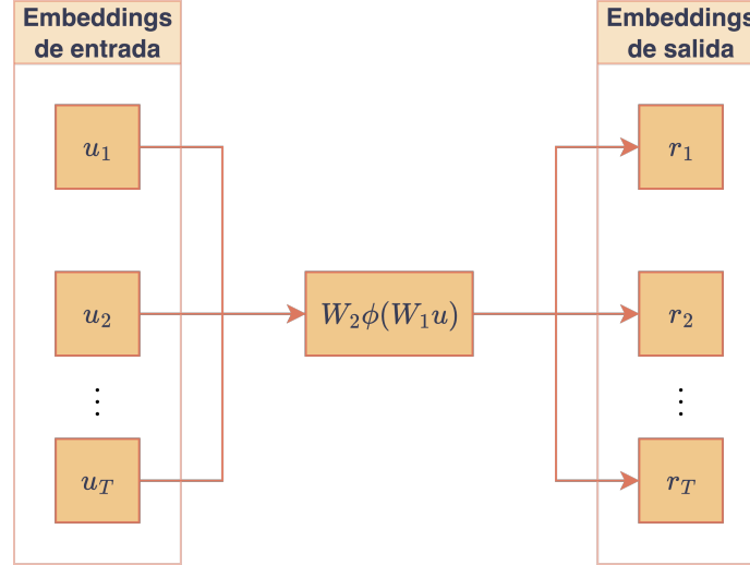
Figura 47: Diagrama de la red feedforward aplicada de forma independiente a cada embedding de la secuencia.
