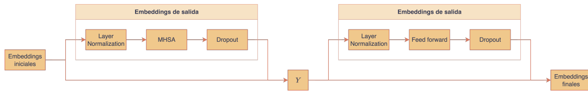
Figura 48: Diagrama de un bloque Transformer con self-attention multicabezal, red feed-forward, layer normalization, dropout y conexiones residuales.
