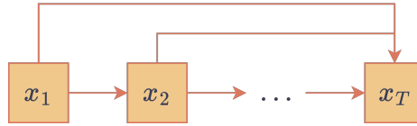
Figura 30: DAG asociado a un modelo autorregresivo.
