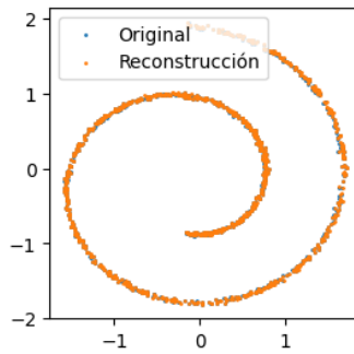
Figura 73: Reconstrucción realizada por un autoencoder clásico.
